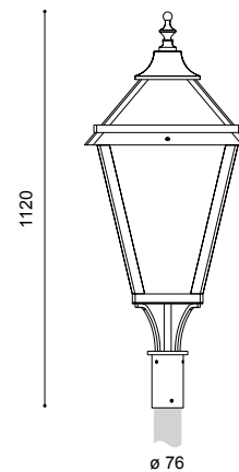
\varnothing 76
