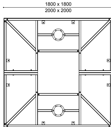
Unterkonstruktion UQ XII/2
