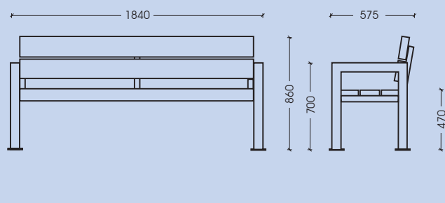
Petra B Q I with flange plate con flangia 86 kg
