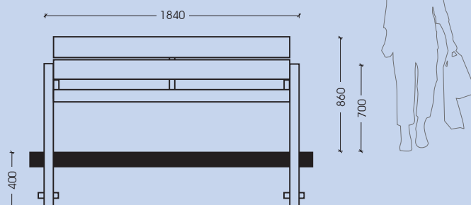
with root con tubo da interrare 92 kg
